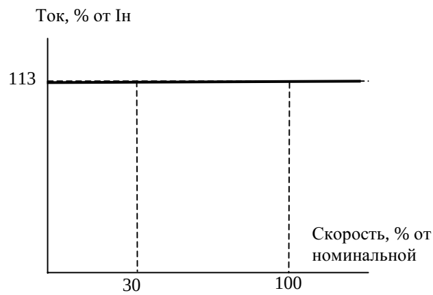
Вентиляторная нагрузка (9-10 = 1)
