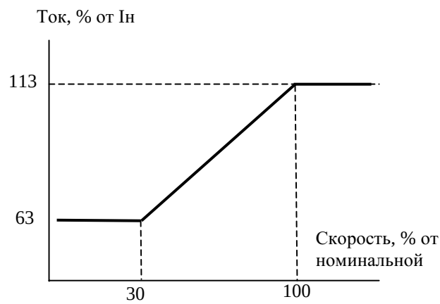
Вентиляторная нагрузка (9-10 = 1)
