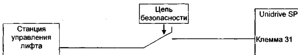
Рис. 5. Аппаратная блокировка сигнала разрешения работы привода
