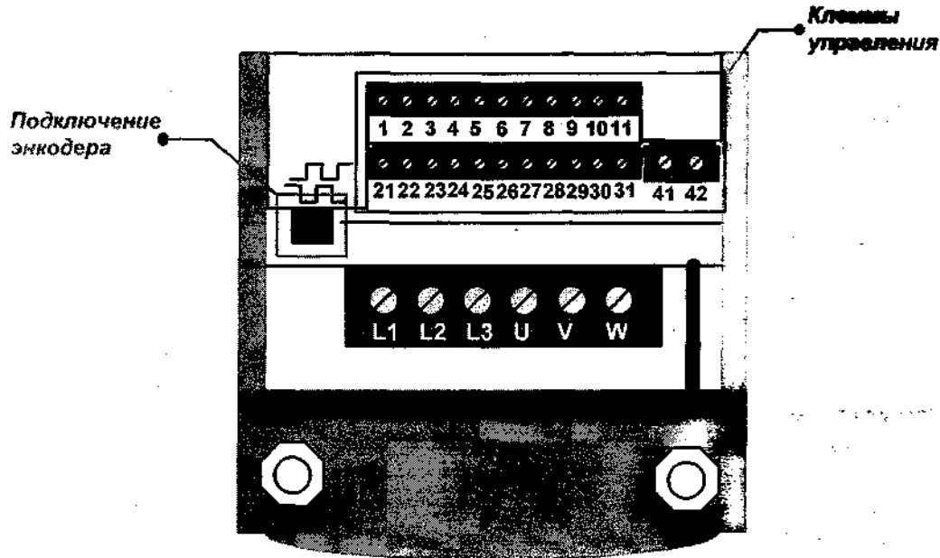
Рис. 2. Клеммы управления и разъем подключения энкодера привода
