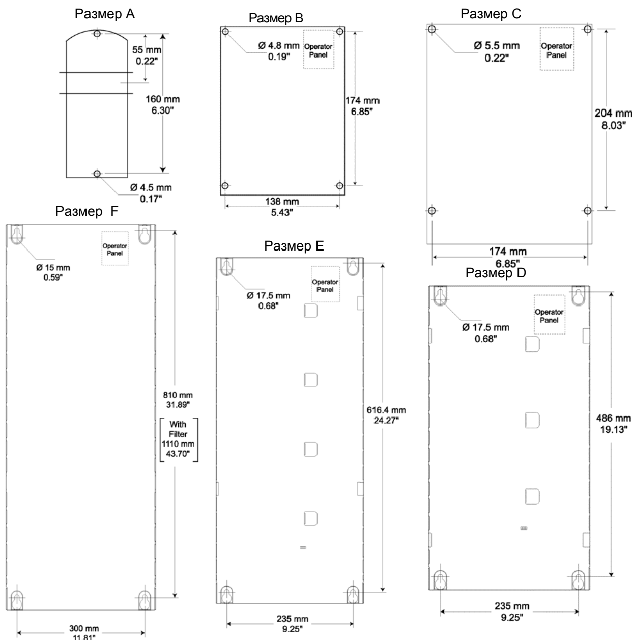
Рисунок 2-1. Габаритные размеры COMBIDRIVE 4
