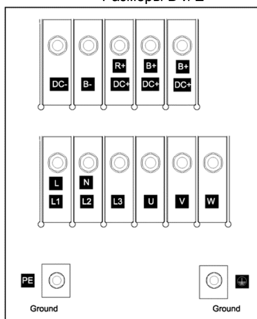
Рисунок 2-2. COMBIDRIVE4 - клеммы силовых присоединений
