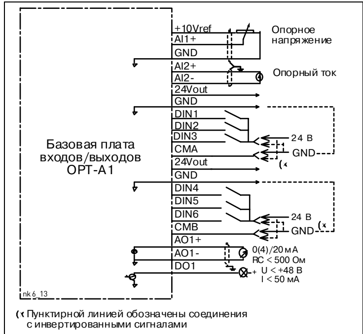
Рисунок 6-24. Принципиальная схема подсоединения базовой платы входов/выходов (OPT-A1)
