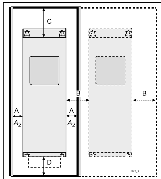
Рисунок 5-11. Вентиляционные промежутки
