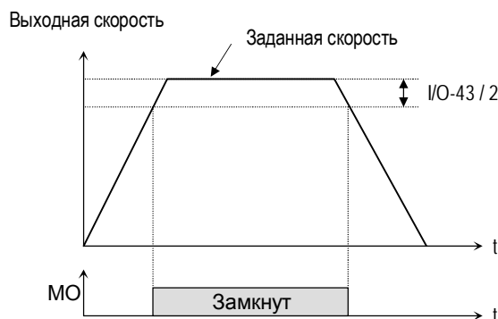
[МО, установка «Финд-1»]
