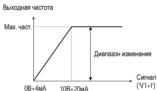
[Источник задания скорости: “V1+I”]
