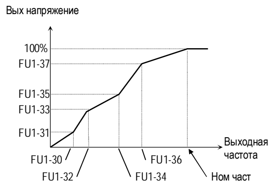
[Специальная U/F-характеристика]
