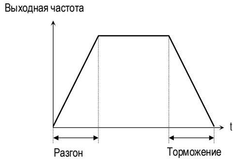
[Линейная характеристика разгона/торможения]
