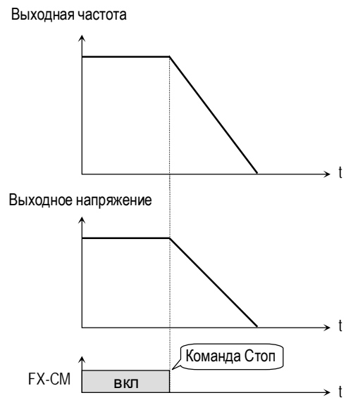
[Тип торможения: «Торм»]
