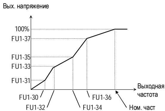
[U/F-характеристика пользователя]
