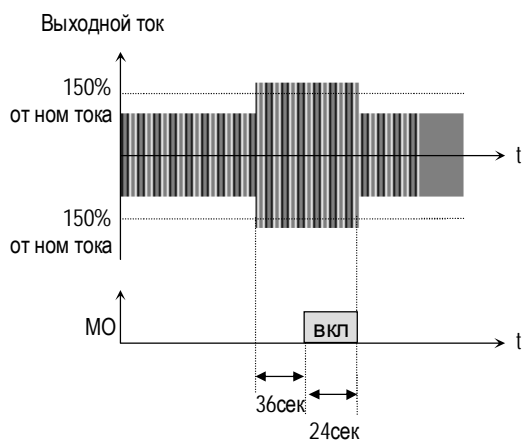
[МО, установка «Перегр I»]
