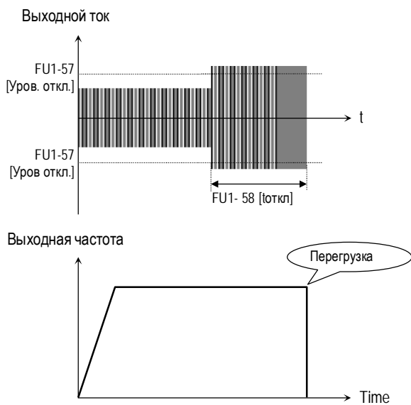
[Отключение при перегрузке]
