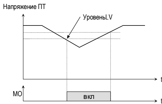
[МО, установка «LV»]
