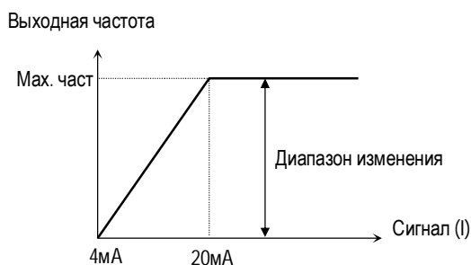
[Источник задания скорости: “I”]
