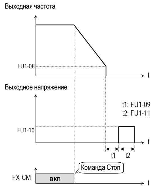
[Тип торможения: «Торм. ПТ»]
