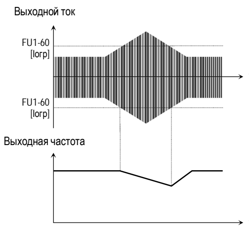
[Токоограничение при постоянной скорости]
