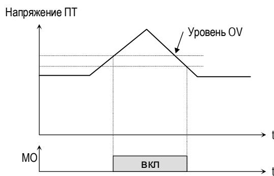
[МО, установка «Перенапряжение»]
