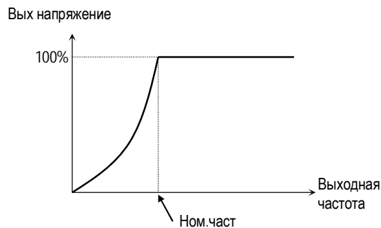
[Квадратичная U/F-характеристика]
