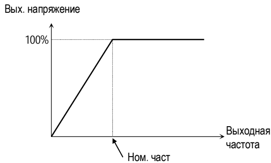
[Линейная U/F-характеристика]
