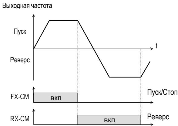
[Тип стартовых команд: "Fx/Rx-1"]
