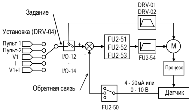
[Структура ПИД-регулятора]
