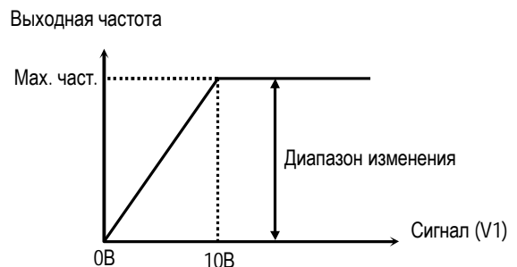
[Источник задания скорости: "V1"]
