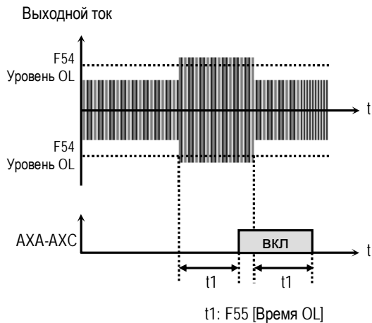
[Сигнал токовой перегрузки]
