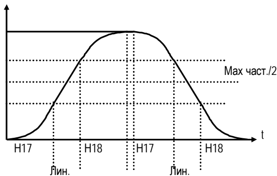
[Настройка S-характеристики]
