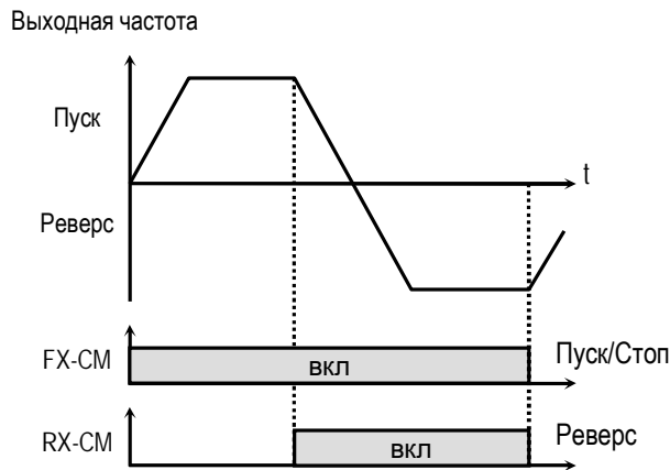
[Тип стартовых команд: "Fх/Rх-2"]
