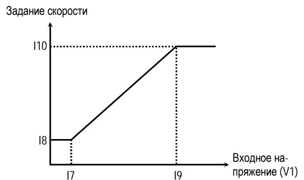
[Зависимость задания скорости от входного напряжения V1 (от 0 до 10В)]
