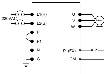
Схема подключения
