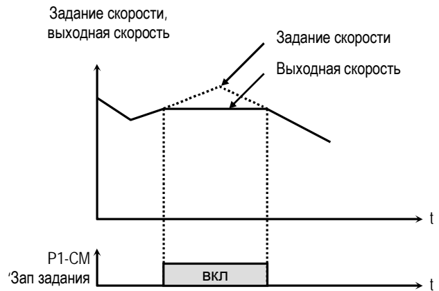
[Режим фиксации выходной частоты]
