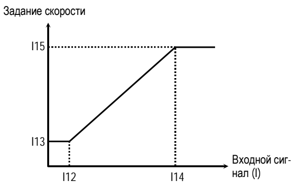
[Зависимость задания скорости от входного сигнала I (от 4 до 20мА)]
