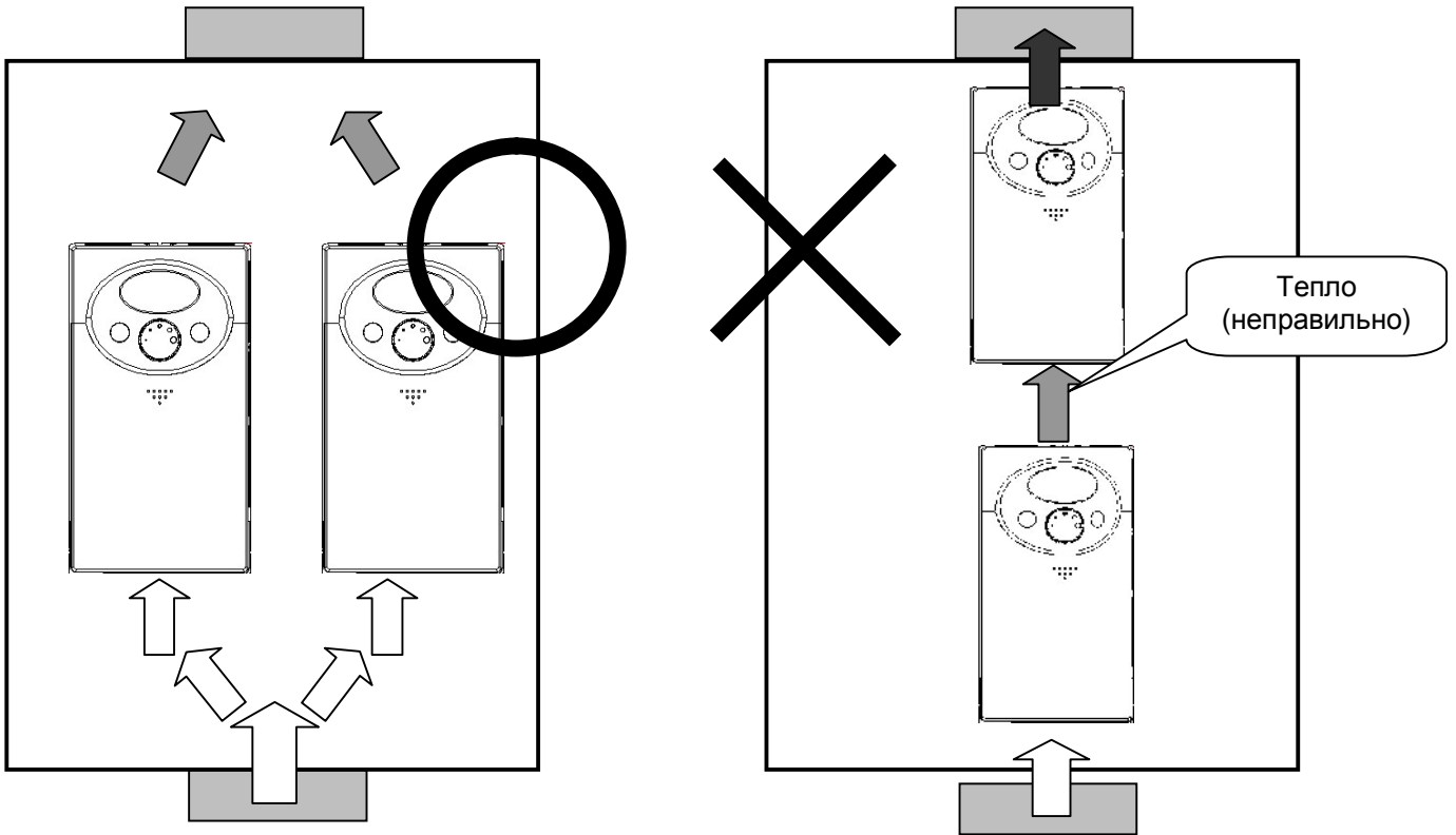
< Установка преобразователей в шкафу >
