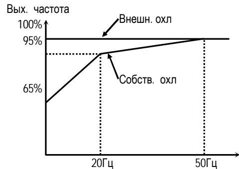
[Характеристика допустимого тока перегрузки]
