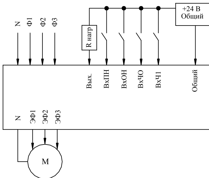
Рис. 2. Блок-схема подключения внешних контактов.
