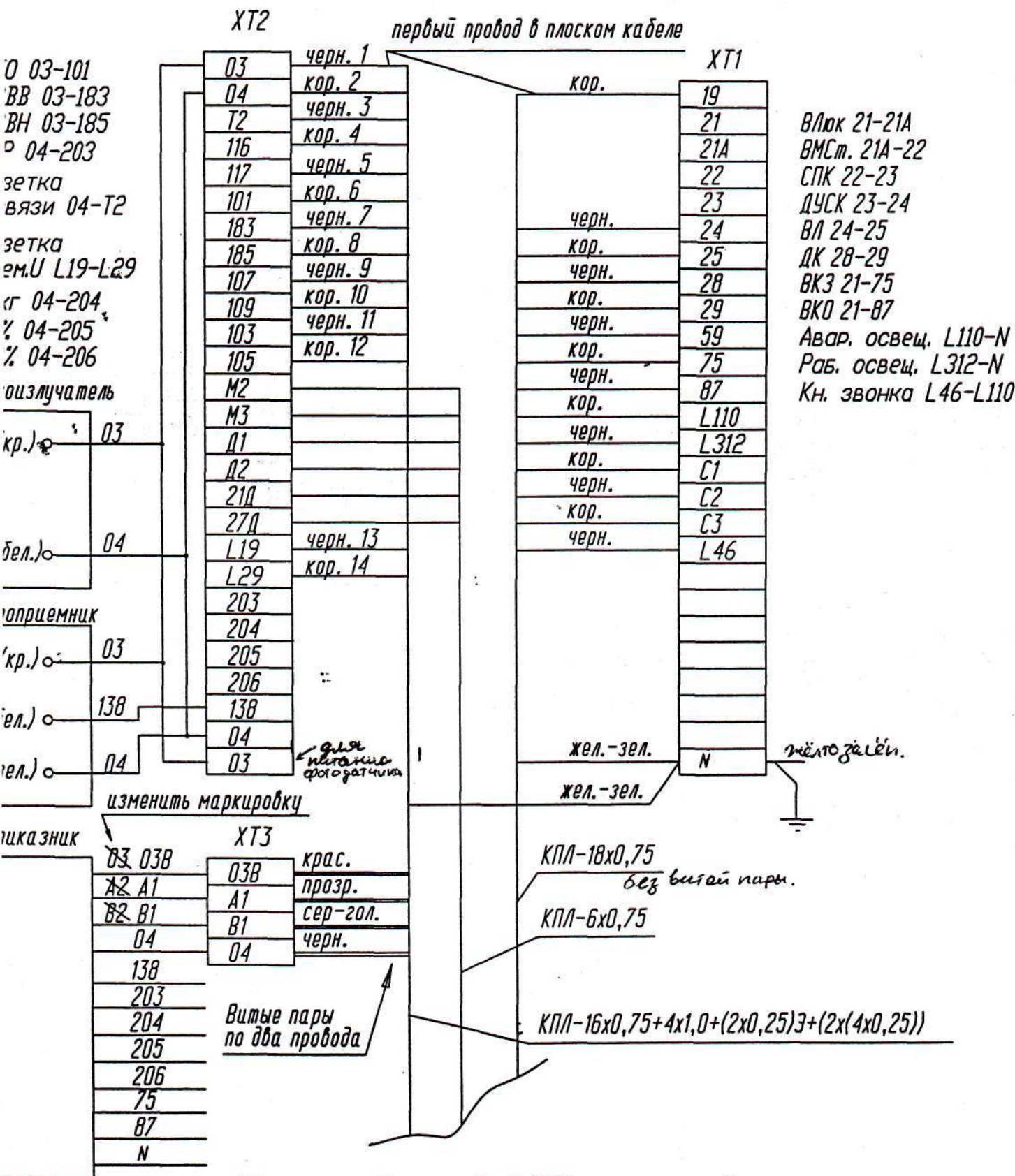
Подключение подвесных кабелей (КПЛ) к клемникам кабины
